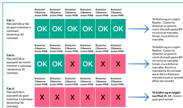
Fíor 9: Loighic Mharcála le haghaidh roghnú COD Praghsála Éagothroime mar thoradh ar Mod_19_19.
